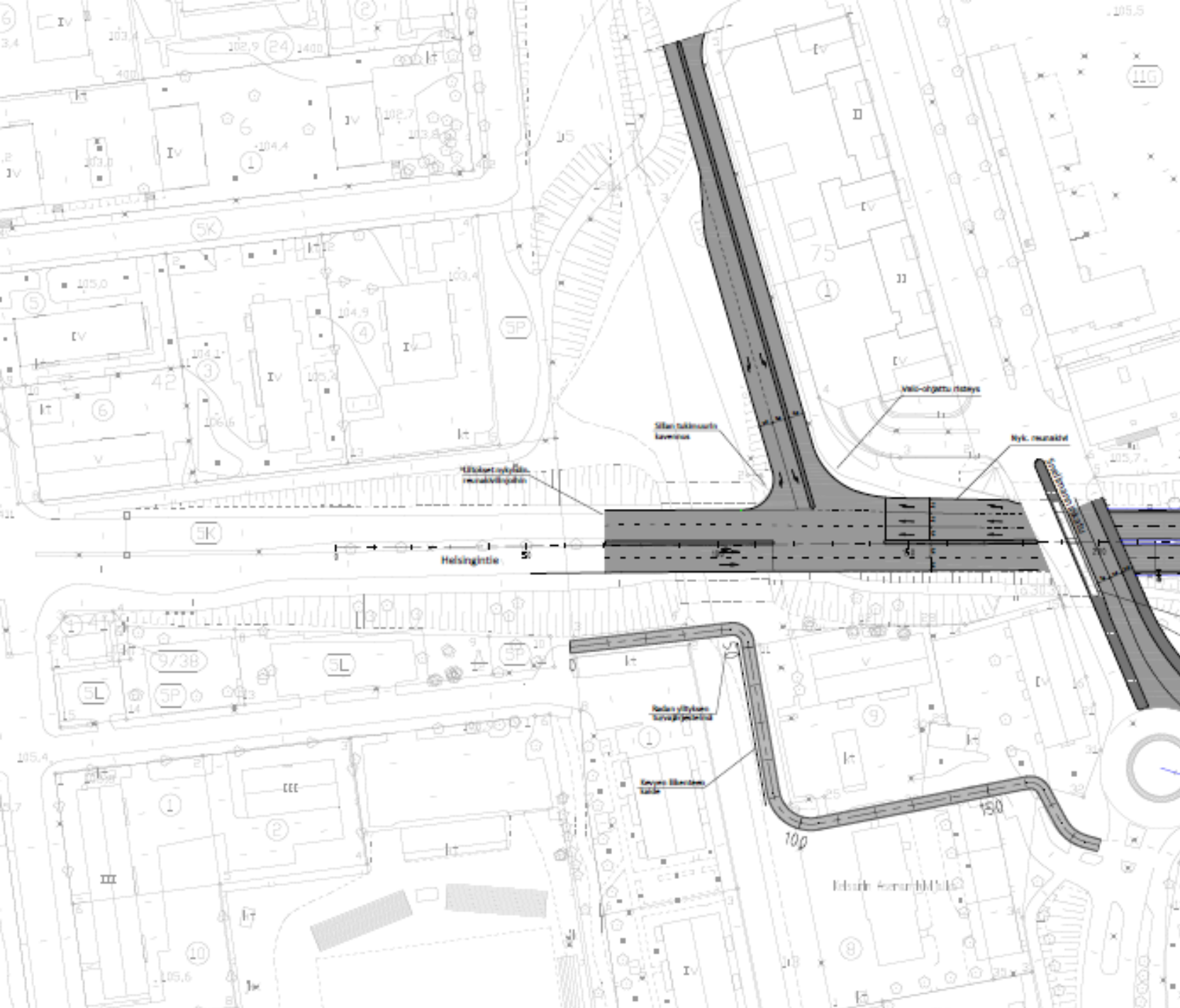
Luonnos liittymän katusuunnitelmasta.
