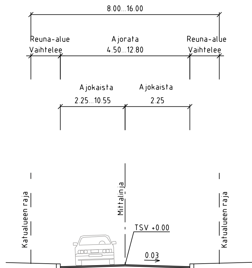
TYYPPIPOIKKILEIKKAUS A-A 1:100
