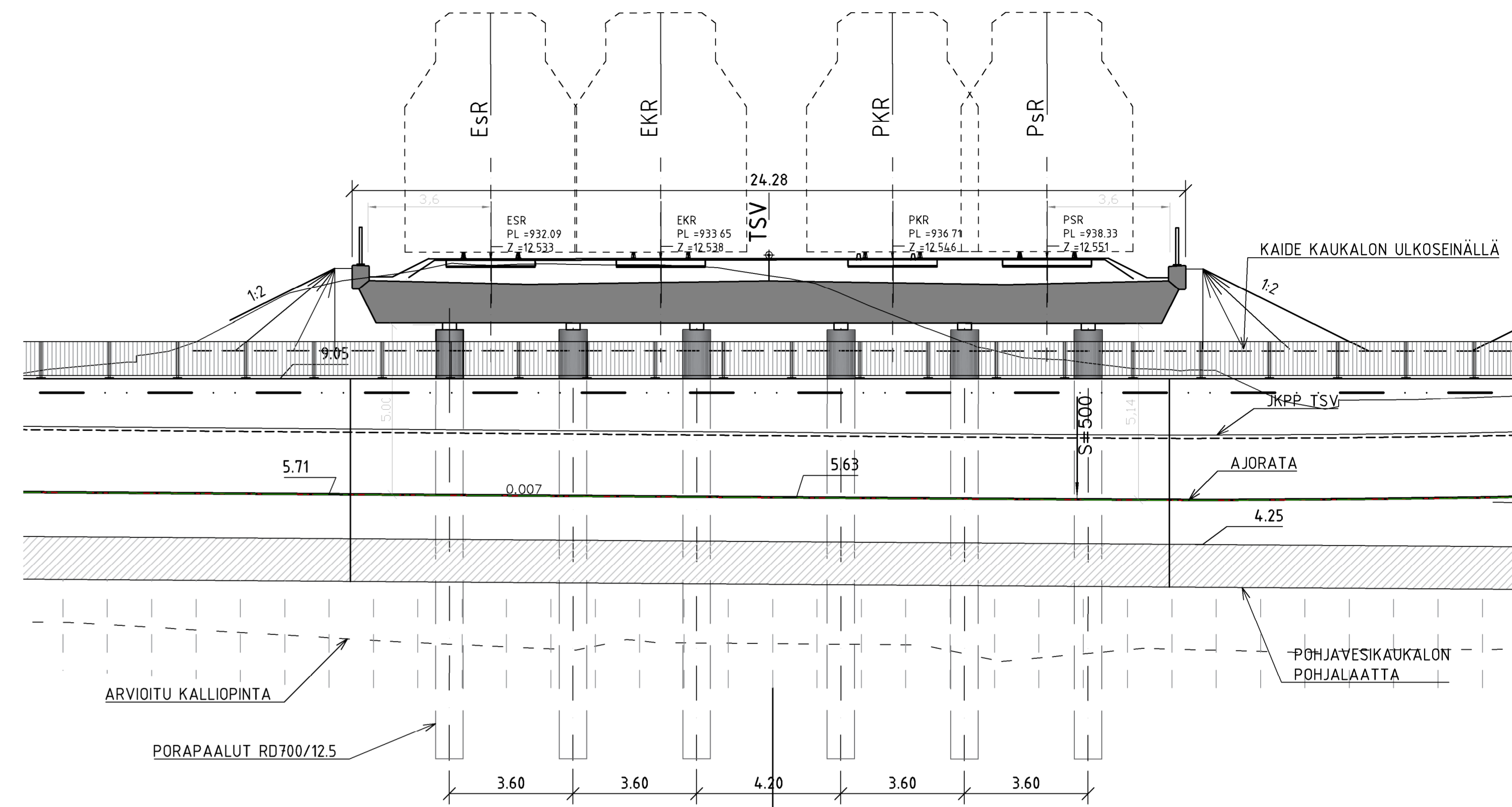
POIKKILEIKKAUS A-A 1:100
