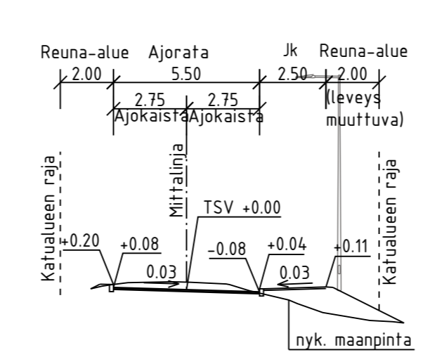
TYYPPIPOIKKILEIKKAUS D-D 1:200
