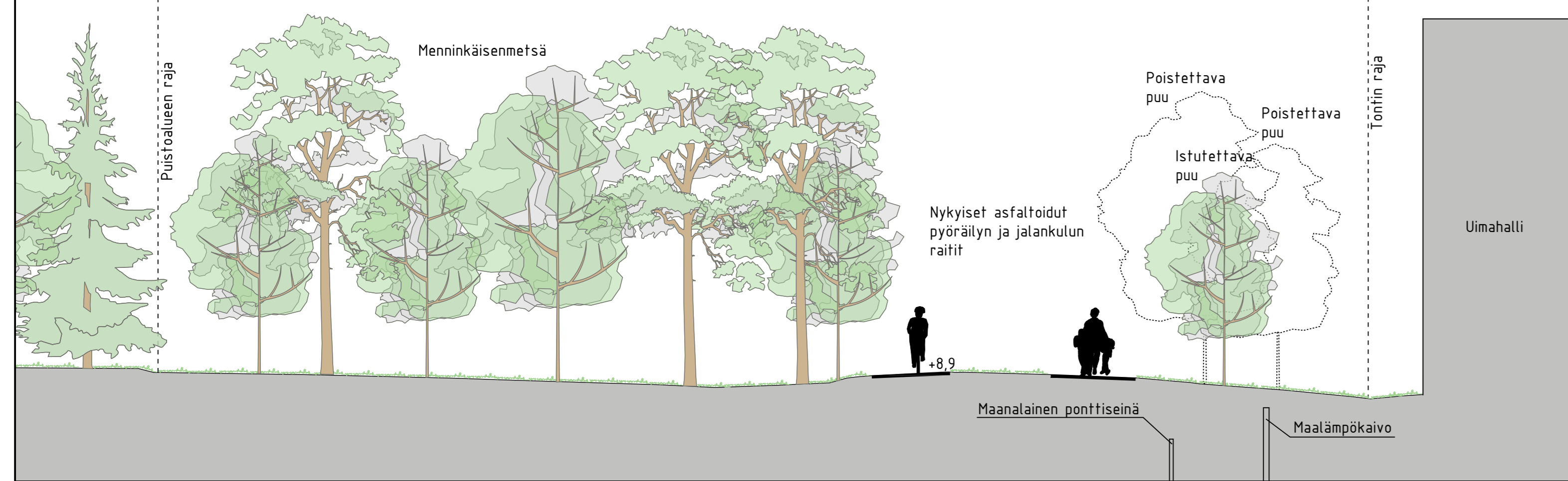
LEIKKAUS A-A 1:100
