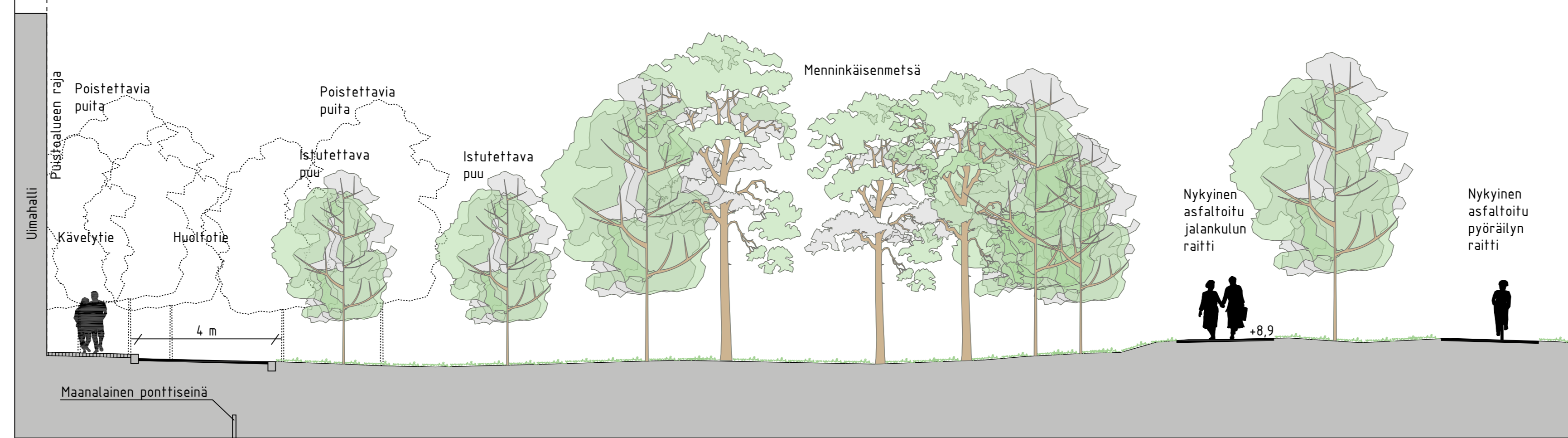
LEIKKAUS B-B 1:100
