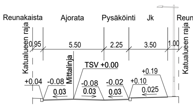
TYYPPIPOIKKILEIKKAUS B-B 1:200
