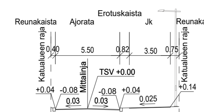
TYYPPIPOIKKILEIKKAUS A-A 1:200
