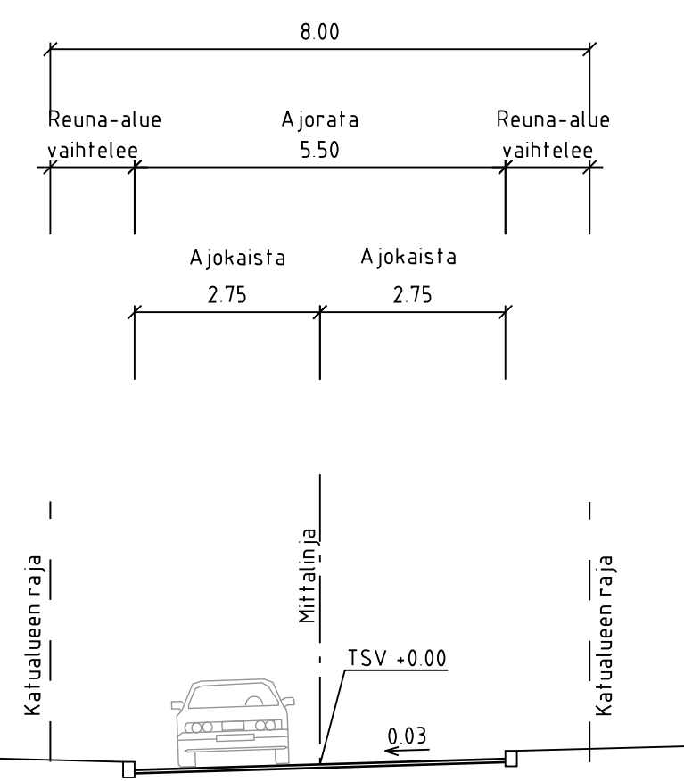
TYYPPIPOIKKILEIKKAUS A-A 1:100
