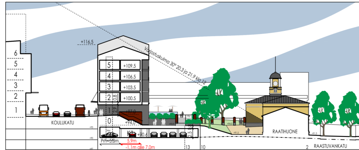
Periaateleikkaus Raatihuoneen korttelin kohdalta.
