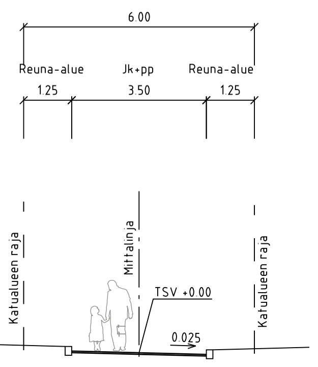
TYYPPIPOIKKILEIKKAUS B-B 1:100
