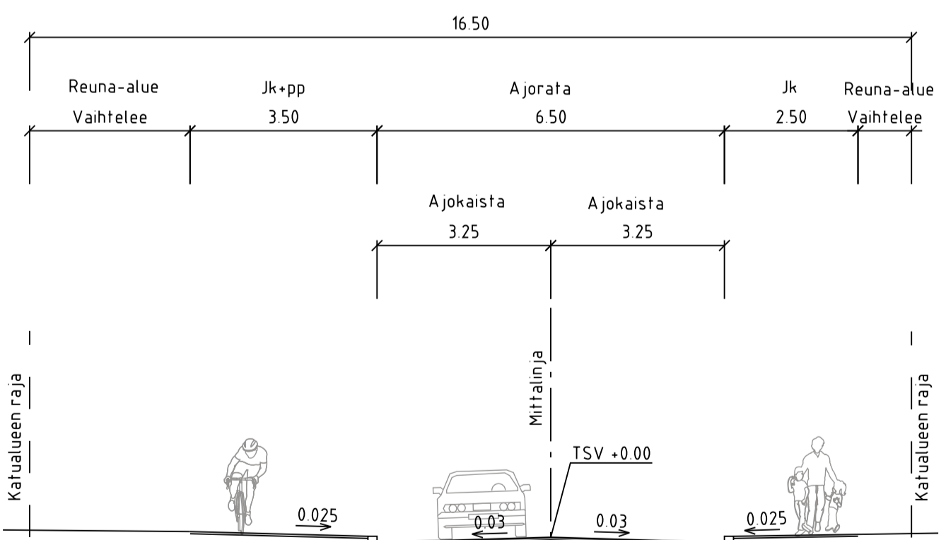
TYYPPIPOIKKILEIKKAUS B-B 1:100
